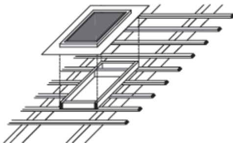
Ovenlys på lægteplanet.
