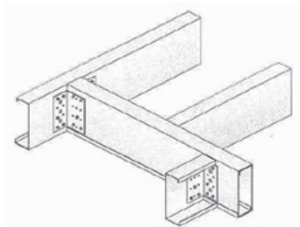
Brug evt. dobbelt C-profil, hvis udvekslingsprofilerne skal bære C-profiler i begge retninger.
